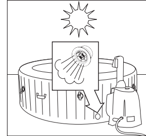
Lucht zet uit in de middaghitte (door warmte). Ontluchtingsventiel laat het overtollige lucht vrij.
